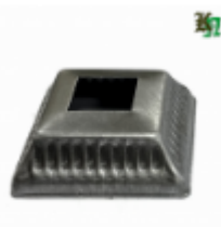
Основание баясины, арт. 8.6020 60x60x1мм, кв.20x20мм Вес: 0.04 кг Цена (за шт): 43 руб.
